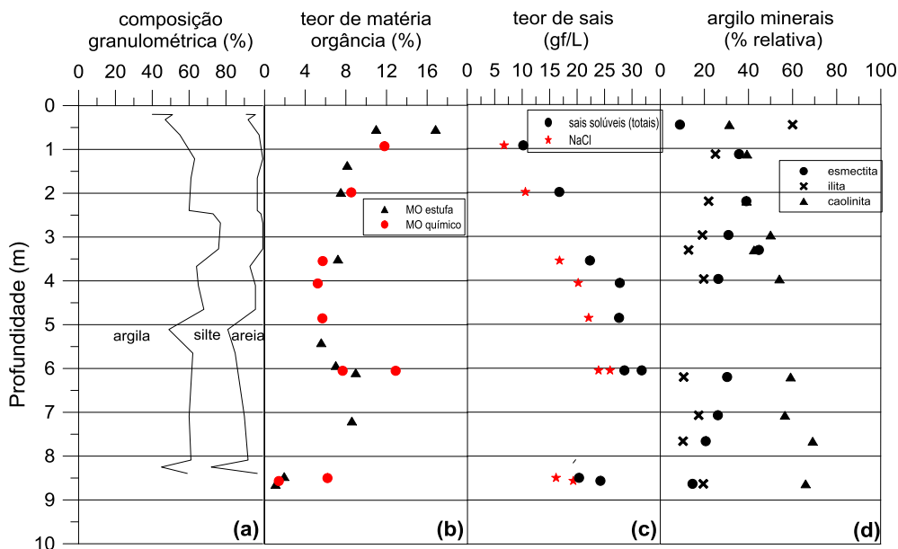
Figura 2. Caracterização geotécnica do depósito de argila muito mole do Sarapuí II: (a) granulometria; (b) teor de matéria orgânica; (c) teor de sais; (d) frações de argilominerais presentes na microestrutura (adaptado de Januzzi et al. , 2015; Danziger et al. , 2015).
