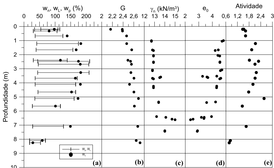
Figura 1. Caracterização geotécnica do depósito de argila muito mole do Sarapuí II (Adaptado de Januzzi et al. , 2012a; Danziger et al. , 2019).
