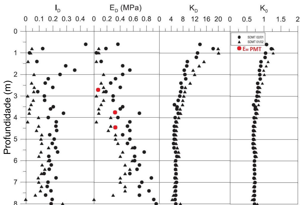
Figura 6. Valores de parâmetros dos ensaios de SDMT e PMT obtidos do depósito de argila orgânica muito mole Sarapuí II (adaptado de Januzzi et al. , 2015).
