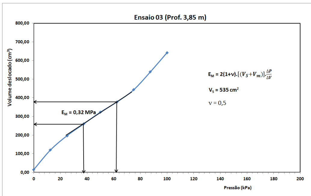
Figura 5. Curva típica de um ensaio com o PMT em depósito de argila orgânica muito mole do Sarapuí II.
