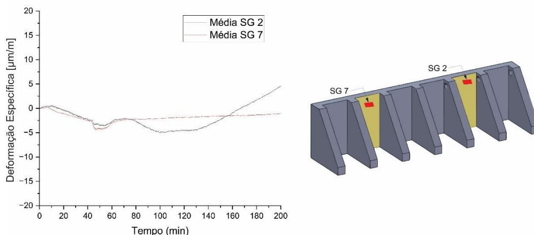
Figura 7. Média da deformação específica na Jusante
