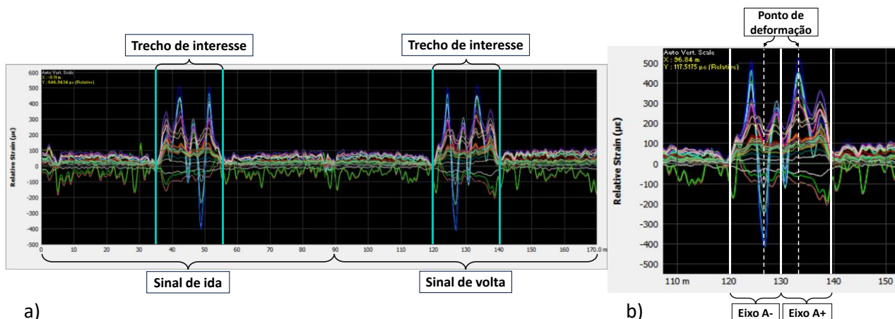
Figura 8. (a) Leitura dos dados no software DITEST Data Viewer da Omnisens. (b) Trecho de interesse.
