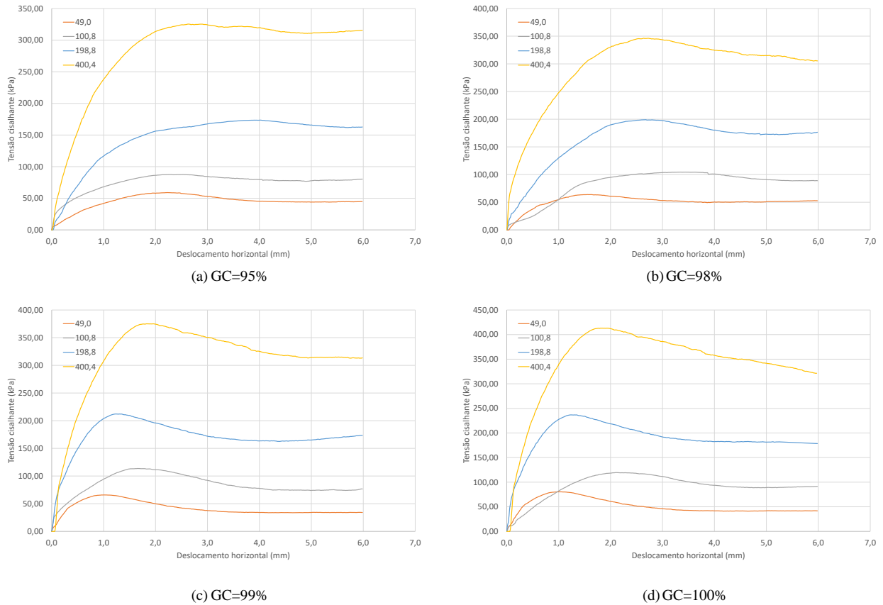
Figura 4. Curvas tensão-deformação em ensaios cisalhamento direto.
