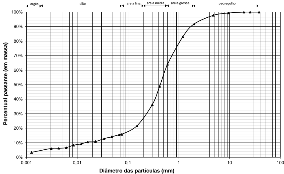
Figura 2. Curva granulométrica do solo estudado
