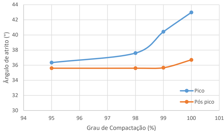
Figura 5. Variações do ângulo de atrito com o grau de compactação.
