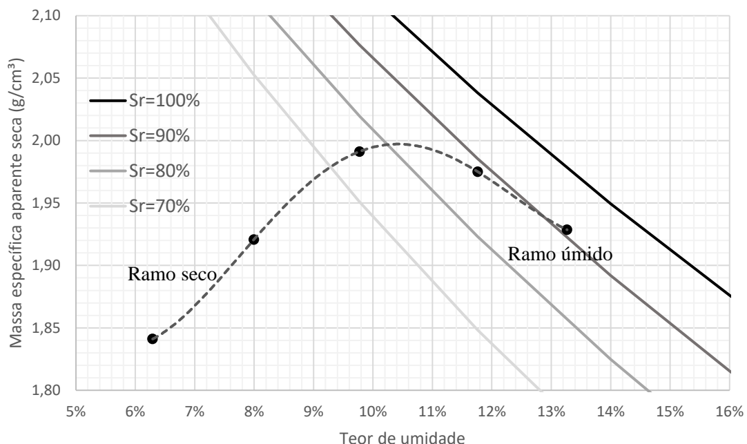
Figura 3. Curva de compactação (Proctor intermediário).
