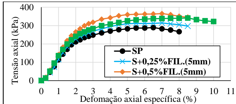
Figura 2: Curvas tensão-deformação obtidas para o solo puro e para as misturas solo-PET filete (filete com comprimento de 5mm). Fonte: Autores (2022).
