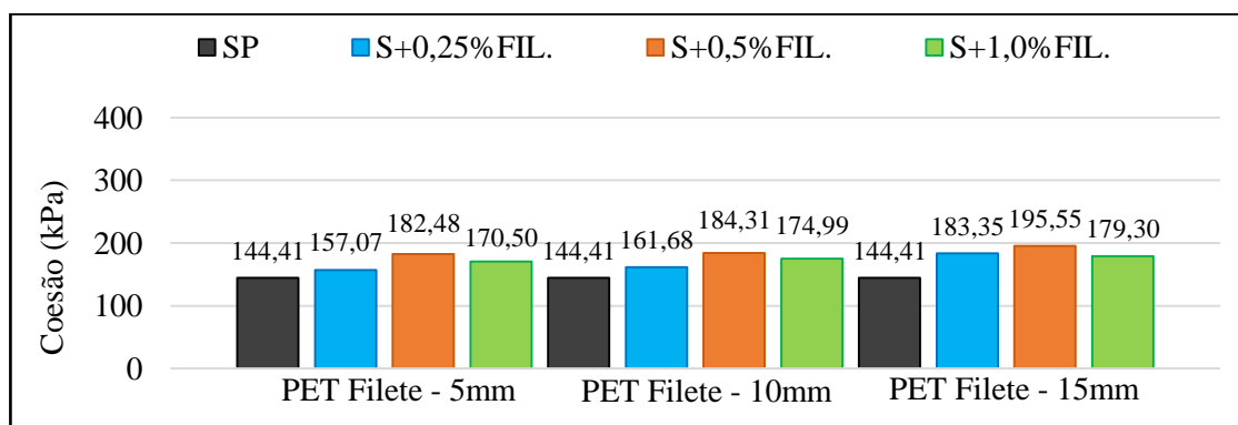
Figura 5: Valores de coesão obtidos para o solo puro e para as misturas Solo-PET filete. Fonte: Autores (2022).
