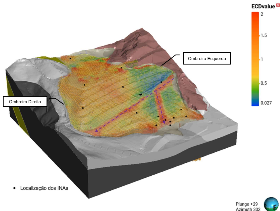
Figura 6. Visão 3D do modelo pedo-litológico incorporado à investigação geofísica.
