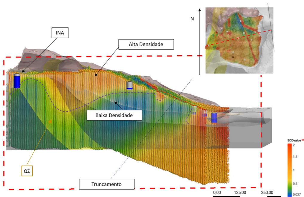
Figura 7. Seção XX' - Comparação dos Indicadores de Nível d'Água e Geofísica.
