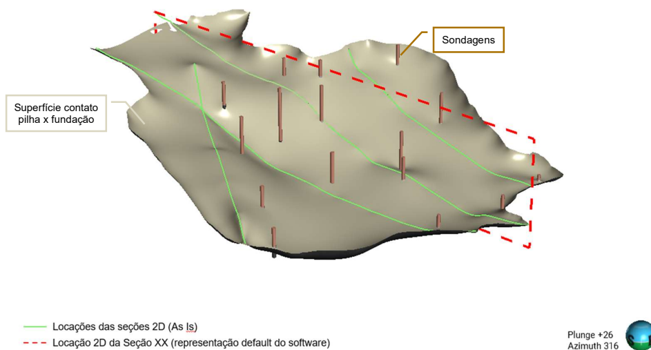
Figura 1. Contato pilha x fundação e inputs
