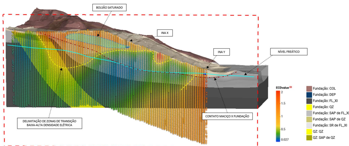
Figura 8. Seção XX' – Representação do bolsão suspenso.
