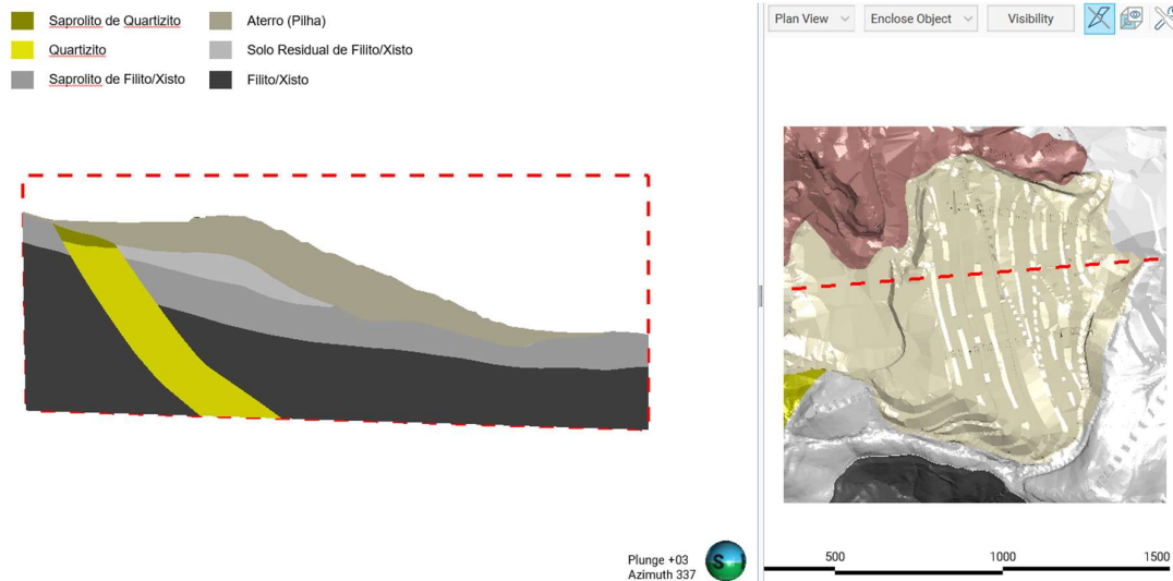
Figura 4. Corte - seção XX' (modelo), sobreposto à seção XX' 2D (As Is) e localização em planta.
