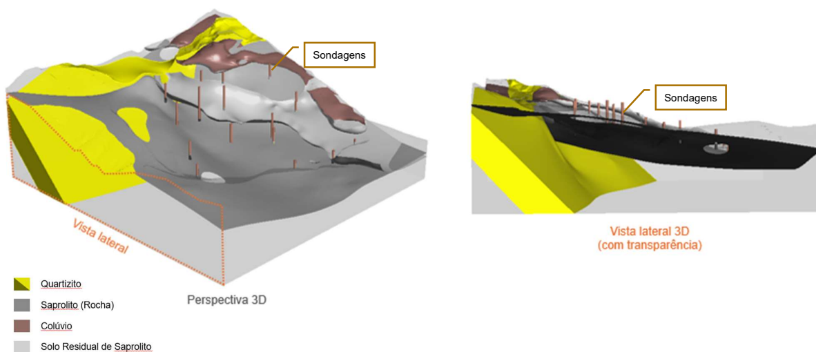
Figura 3. Visão 3D da diferenciação dos elementos constituintes da fundação.
