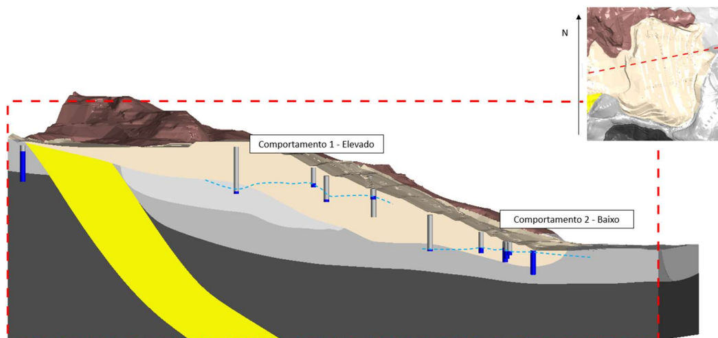
Figura 5. Seção XX' - Comportamentos de níveis d’água internos e localização em planta.
