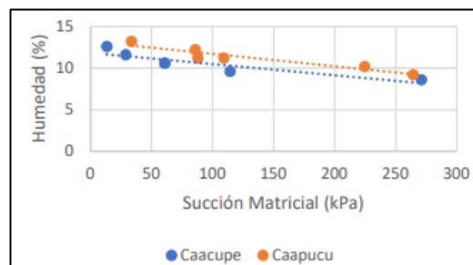
Figura 5. Curva de succión de los suelos estudiados. Fuente: Elaboración Propia.
