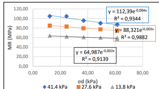
Figura 4. Comportamiento resiliente del suelo de Caacupé en función al esfuerzo. Fuente: Elaboración Propia.
