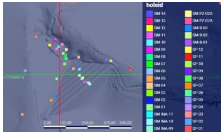
Figura 1. Localização das sondagens consideradas no modelo em planta.
