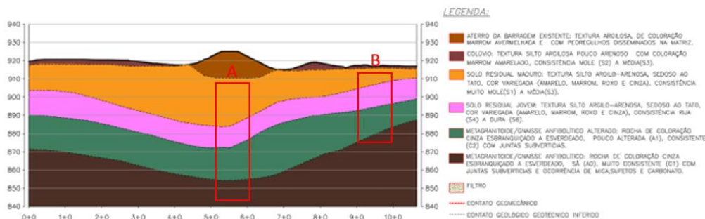
Figura 4. Seção D realizada manualmente por um especialista (Direita) e realizada pelo software Leapfrog Works 2023.1.
